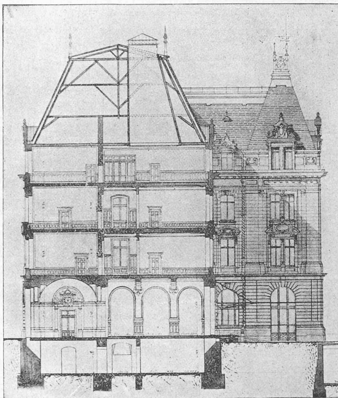
Fig. 4. — Coupe transversale.
