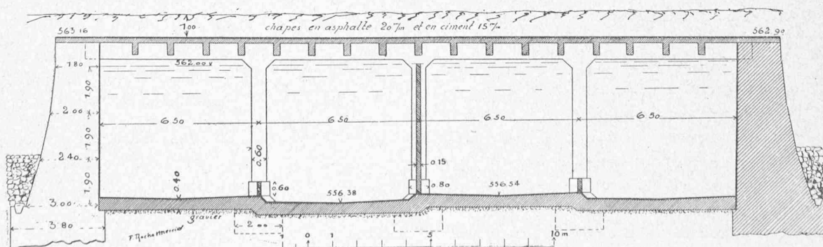
Coupe en travers dans l'axe du réservoir.
