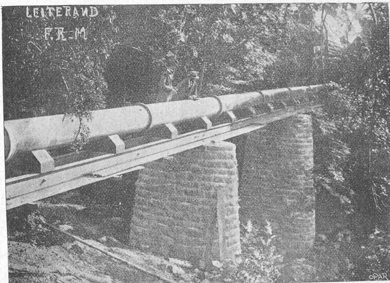
Passerelle sur le Leyterand (St-Légier) avant l'entourage.
