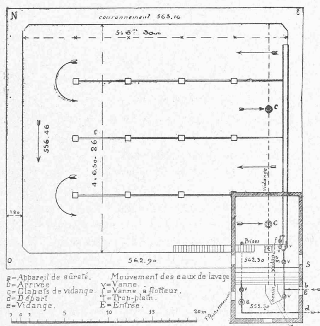
Plan du réservoir.
