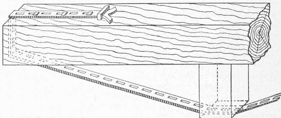
Fig. 18. — Poutre armée.
