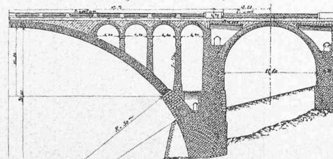
Fig. 9. 1/2 Coupe en long (0,0009)
