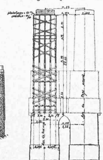
Fig. 10. Coupe du cintre. (dét.)
