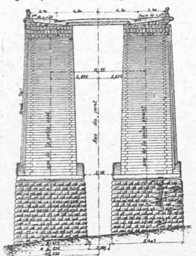
Fig. 6. Coupe en travers l'axe de la grande voûte. (0,00112)
