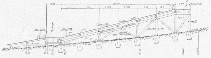
Fig. 5. — Type d'estrade surélevée.
