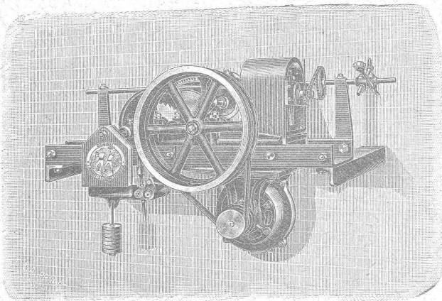
Trebil élévateur pour monte-plats. Système Binkert.
