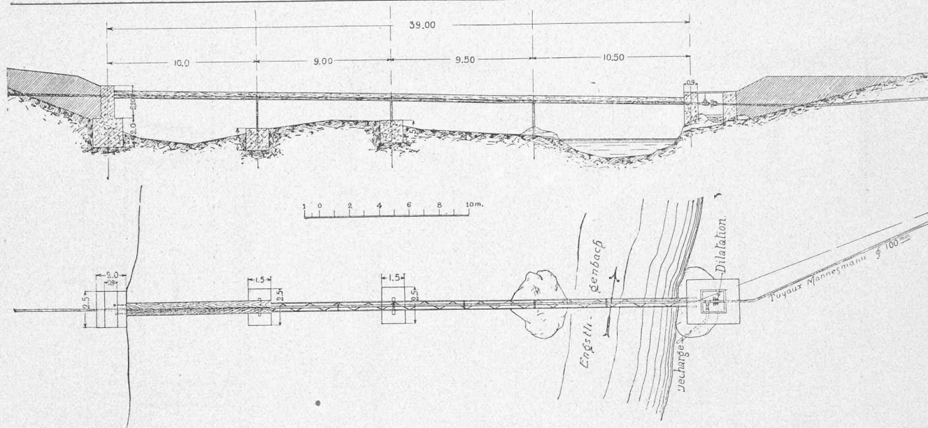
Fig. 16. — Elévation et plan de l'aqueduc sur le ruisseau d'Engstligen.
