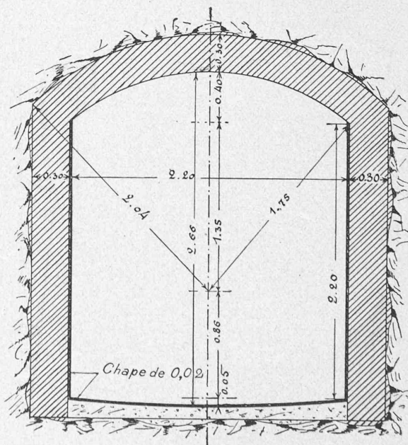
Fig. 11. — Profil-type du tunnel.
