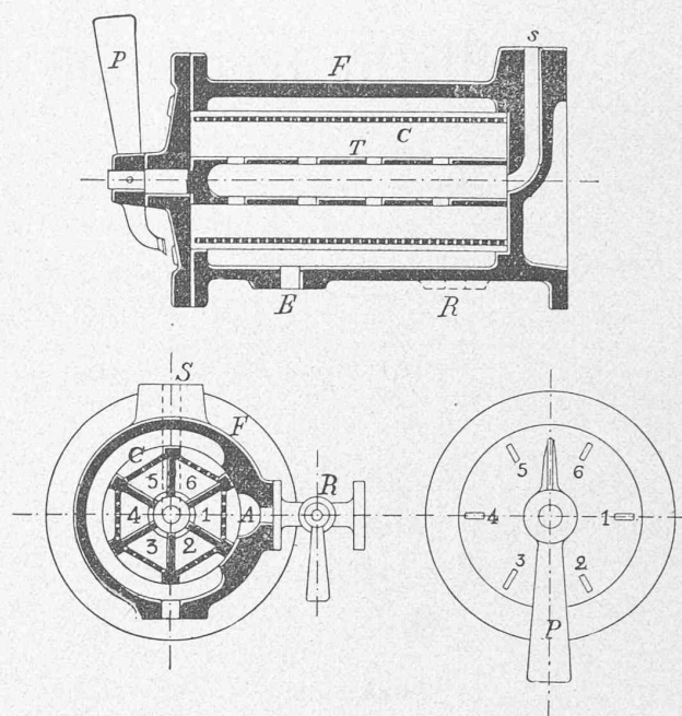
Fig. 22. — Filtre type revolver.
