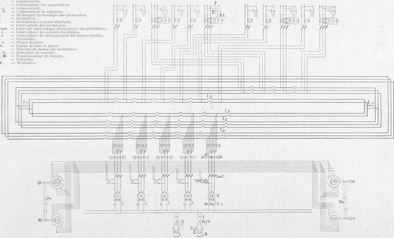
FIG. 33. — SCHEMA GÉNÉRAL DE L'USINE GÉNÉRATRICE DE LA DERNIER
