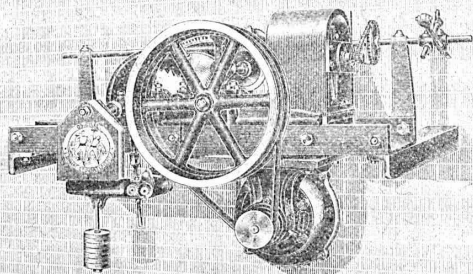
Treuil élévateur pour monte-plats. Système Binkert.
