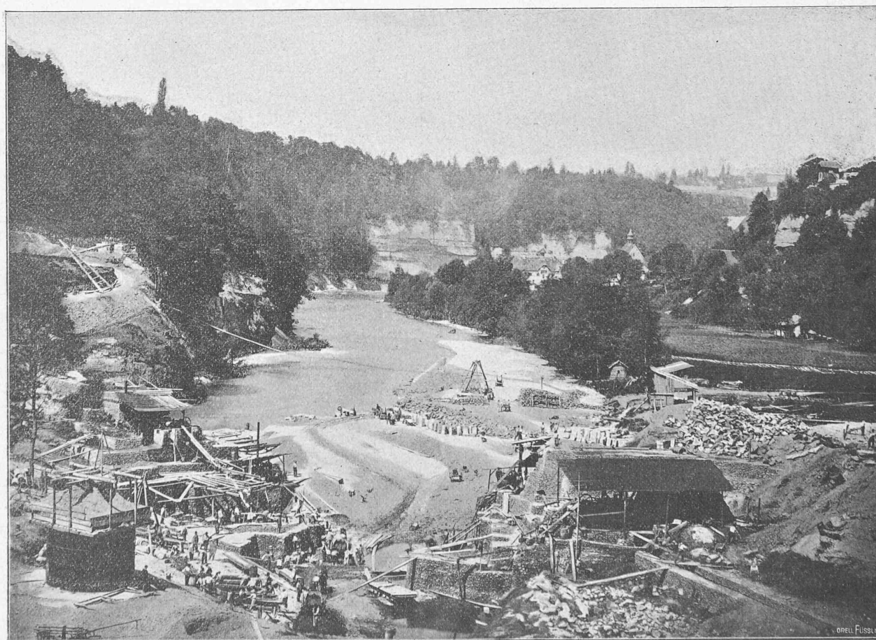
Fig. 3. — Le chantier de l'Usine de la Maigrauge et du barrage sur la Sarine. (Vue prise en 1872.)
