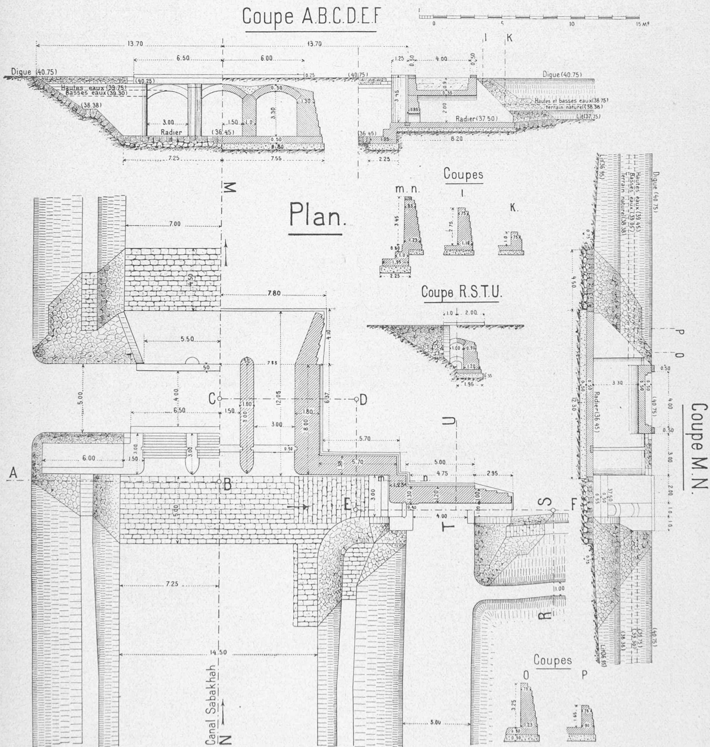
Fig. 16. — Régulateur et prise d'eau (sur la branche Tuah du canal Sabakhah).
