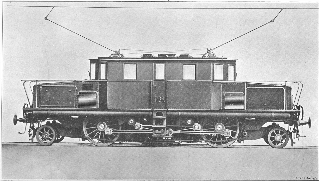
LOCOMOTIVE ÉLECTRIQUE DU SIMPLON Construite par la Société Brown, Boveri & C ie .
