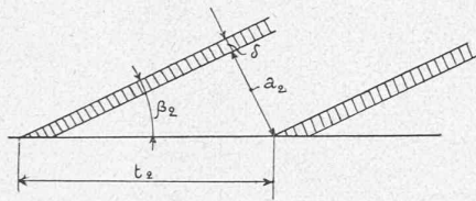
Fig. 7. — Fin d'aubage de turbine axiale.
