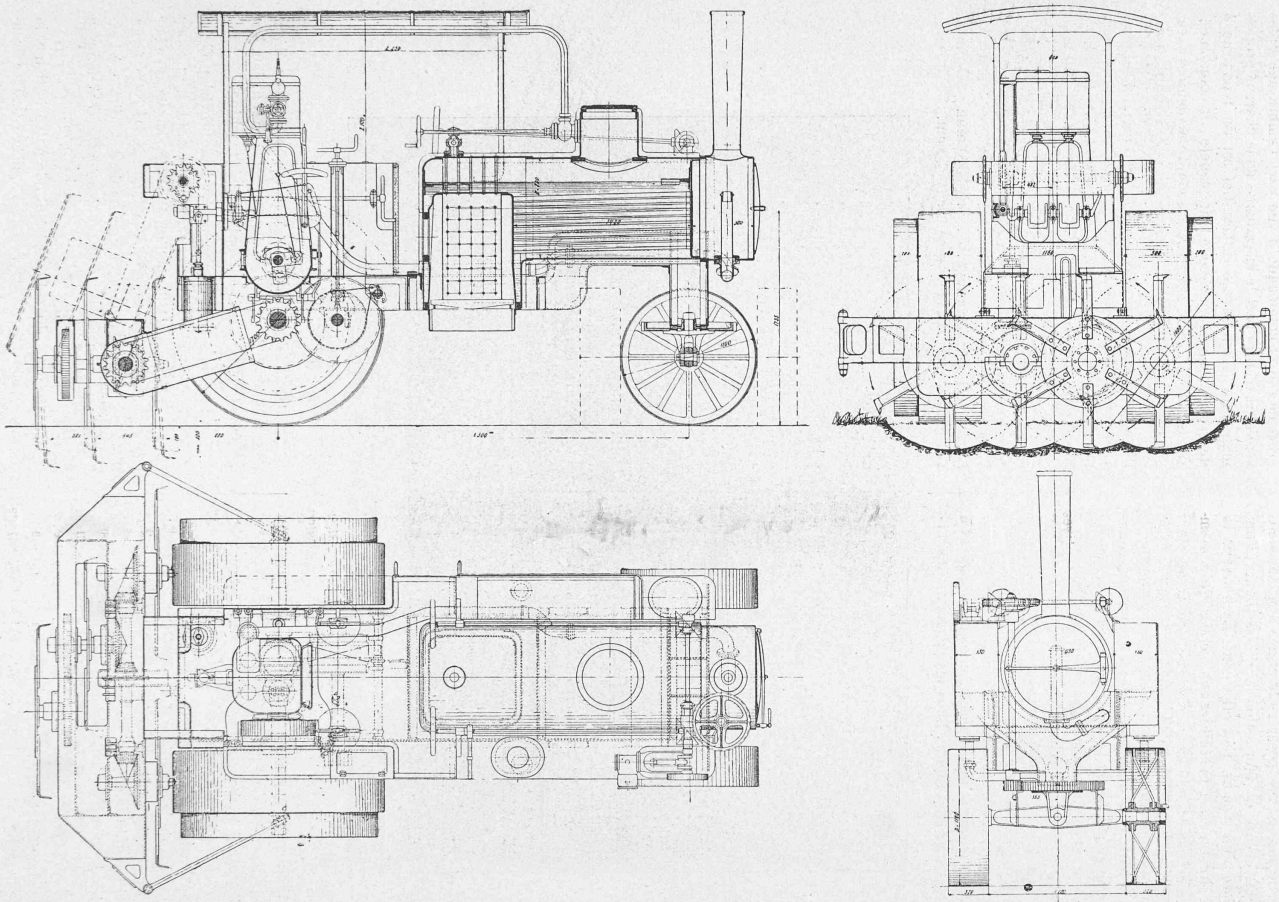
FIG. 3. — LABOUREUSE A VAPEUR (MODELE DE 45 CHEVAUX). — Echelle : 1 : 40.
