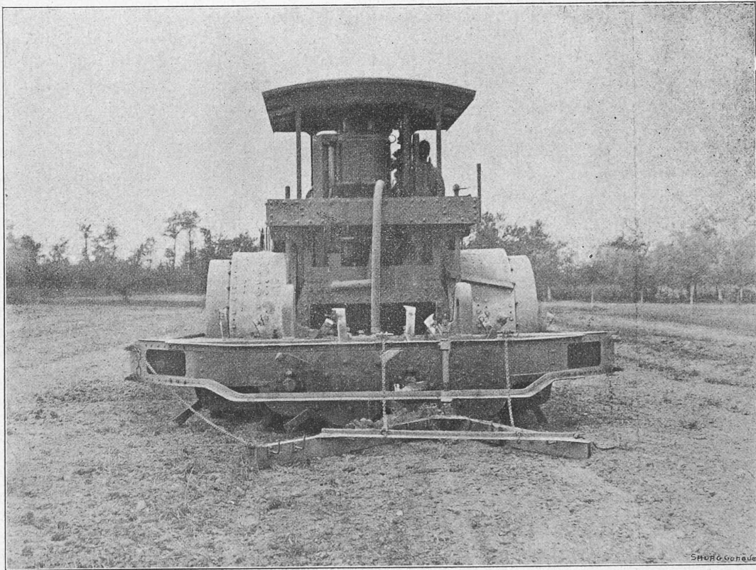
Fig. 2. — Laboureuse à vapeur (modèle de 30 chevaux), avec l'appareil à labourer en service.
