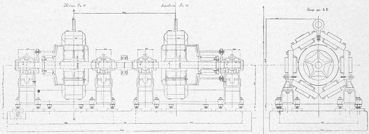
Fig. 21. — Groupe survolteur.
