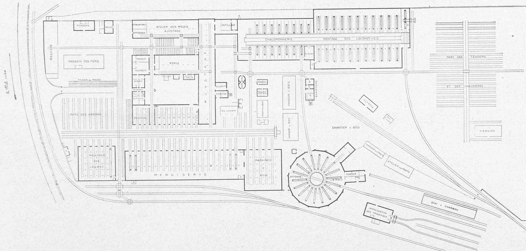
Planche 4. — Plan de situation.
