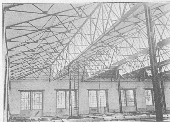
Fig. 13. — Vue intérieure du montage des locomotives. Constructeurs de la charpente métallique Wartmann & Vallette, Brugg.
