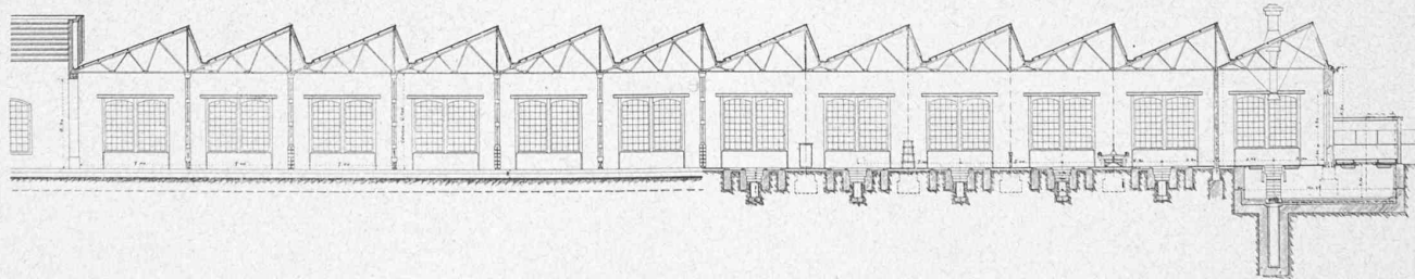
Coupe longitudinale.
