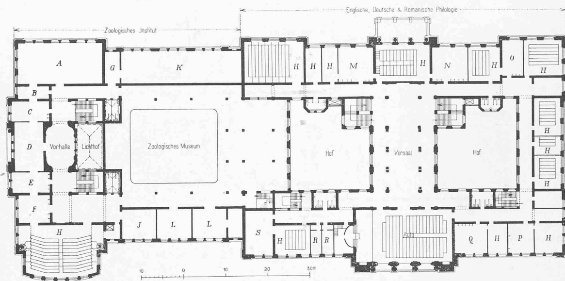
Plan du premier étage. — 1 : 800.
