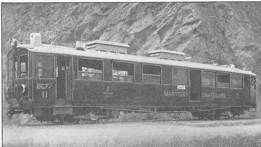
Fig. 39. — Automotrice à 4 moteurs.
