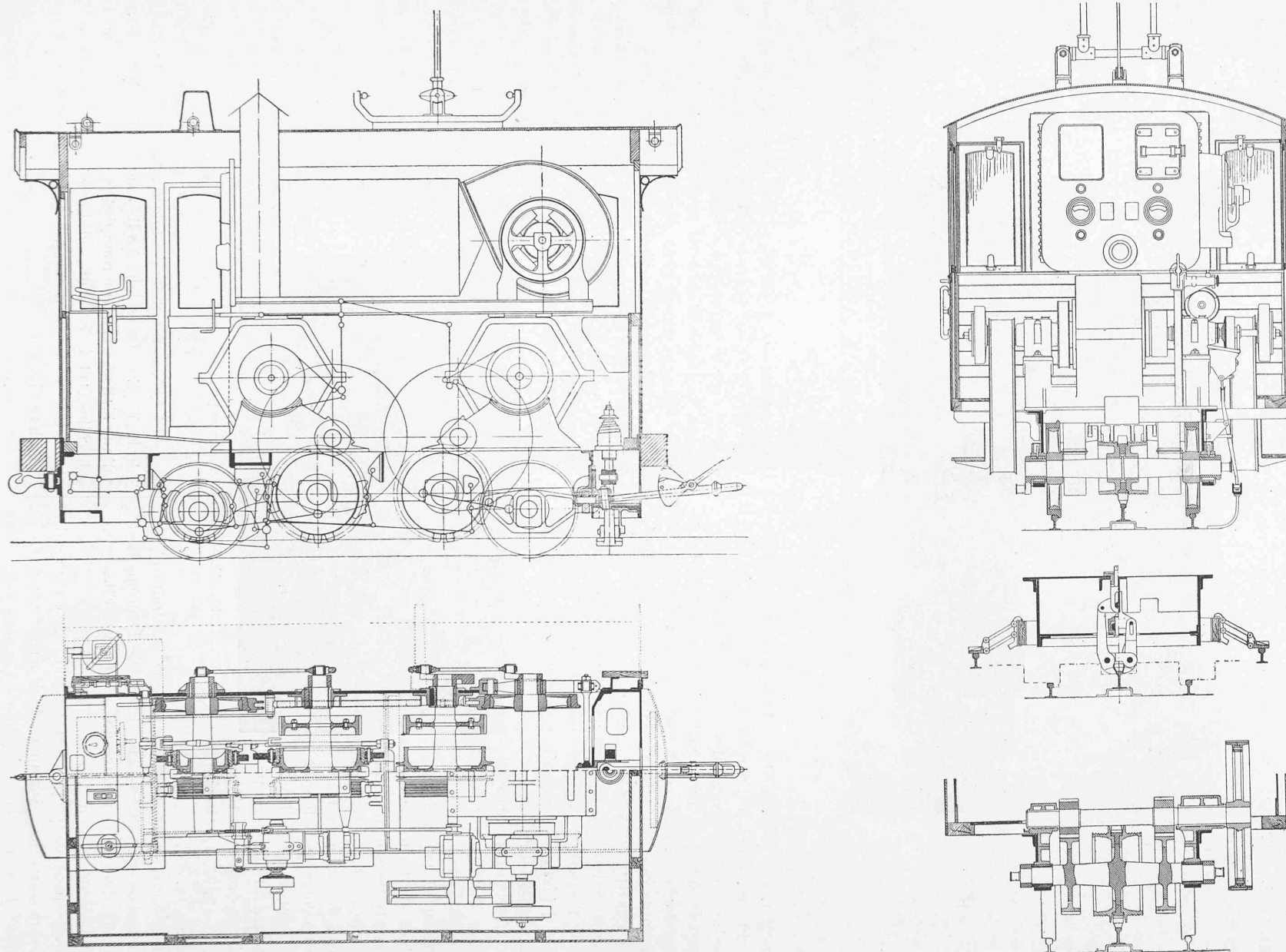
Fig. 45. — Locomotive électrique. — Echelle 1 : 40.
