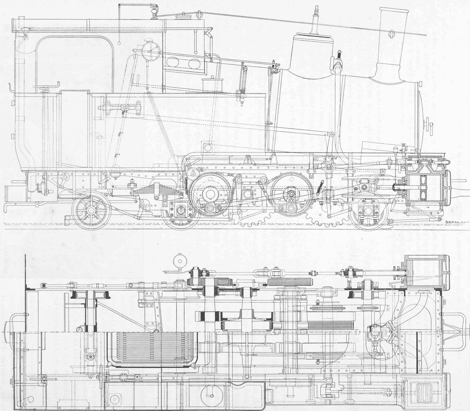
Fig. 18. — Locomotive du chemin de fer de Chamonix au Montanvers. — Echelle 1 : 30.
