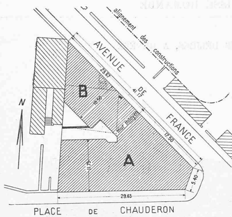
Plan de situation. — 1 : 800.
