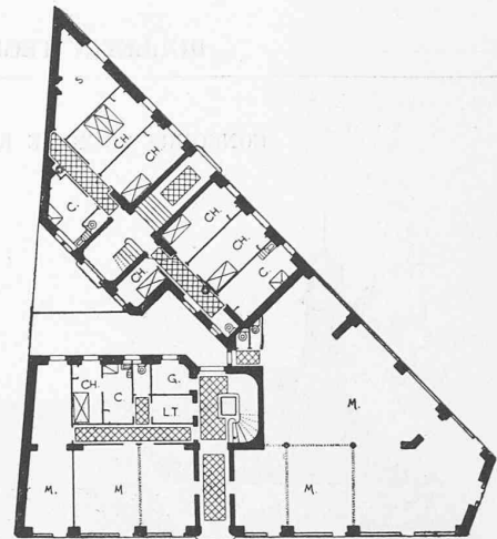
Plan du rez-de-chaussée. — 1 : 500.
