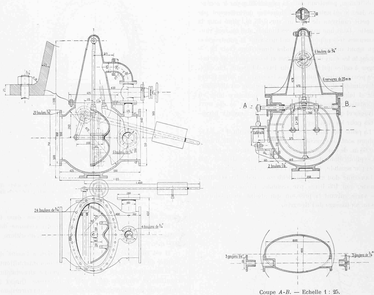
Fig. 4. — Vanne automatique du sûreté placée au départ de la conduite de mise en charge de l'usine de Sonzier.
