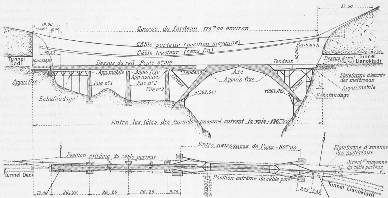
Fig. 4 et 5. — Elévation et plan du viaduc pendant les travaux de montage.
