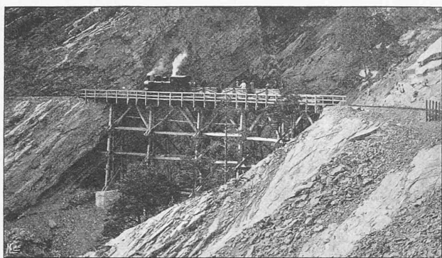
Fig. 27. — Rampe sud. — Pont de service du Luegelkinn.
