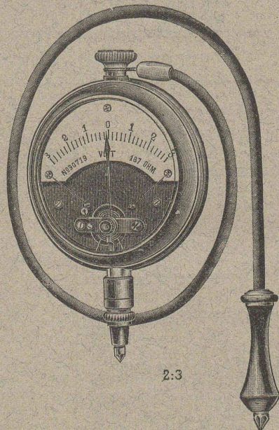
Petit vérificateur apériodique pour accumulateurs, forme de montre.
