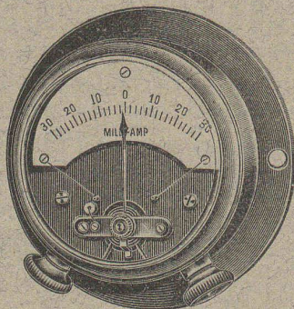
Petit appareil apériodique pour tableau 70 mm. de diamètre.
