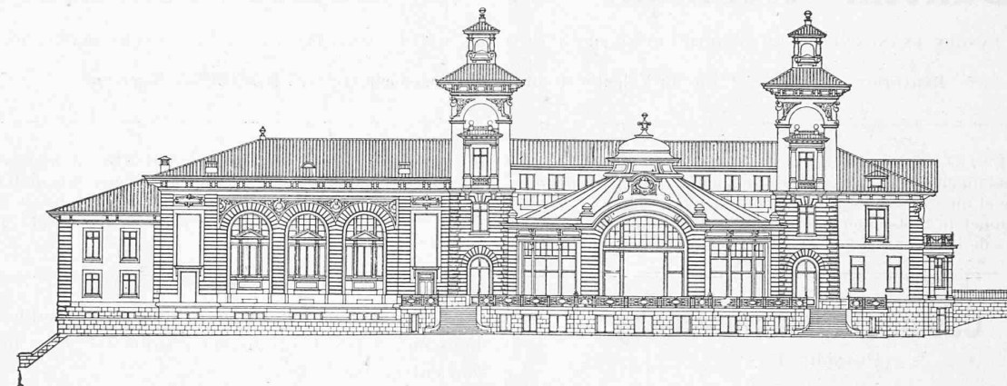
Façade principale. — 1 : 500.
