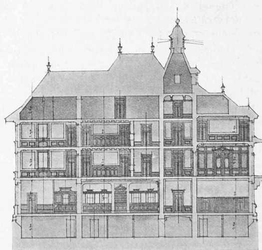
Coupe longitudinale. — 1 : 400.
