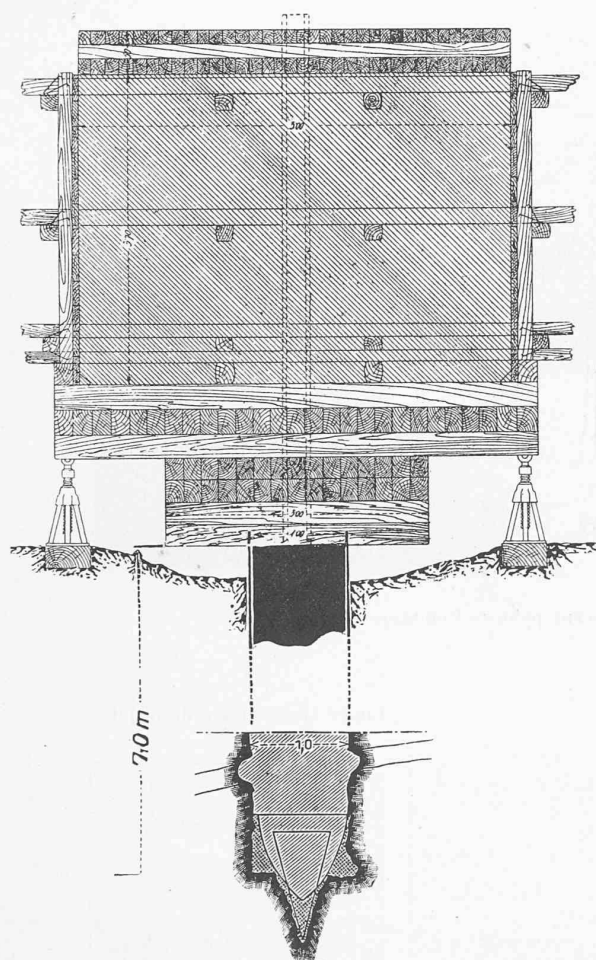
Fig. 6. — Schéma des dispositions de l'expérience de charge directe d'un pylône.
