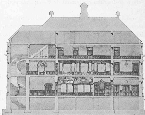
Coupe. — 1 : 400.
