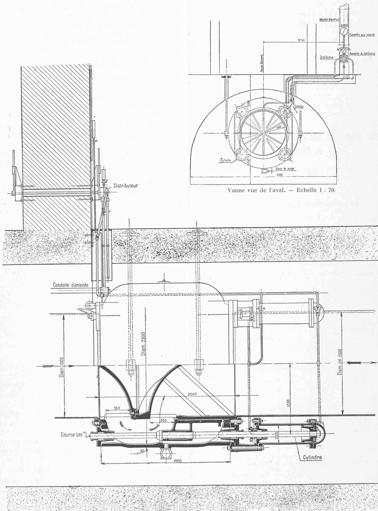
Fig. 17. — Vanne de sûreté de 1,50 m. de diamètre à commande hydraulique.
