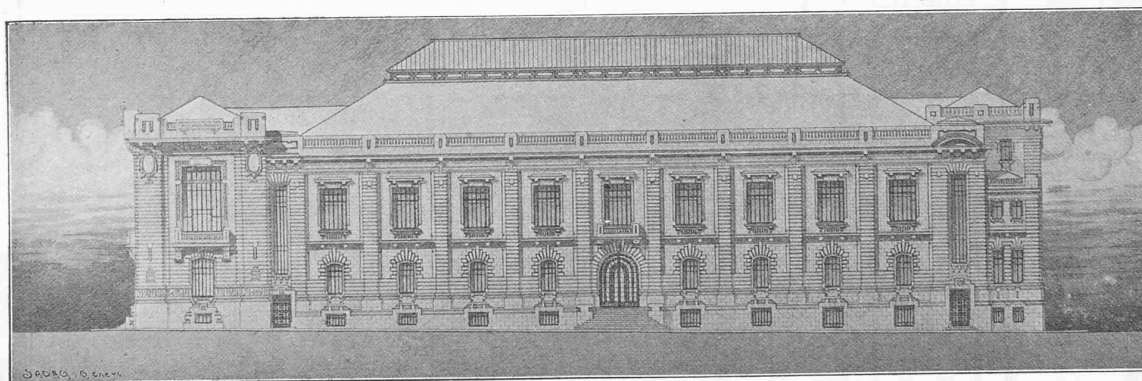
Façade sur la rue de la Plaine. 1 : 600.
