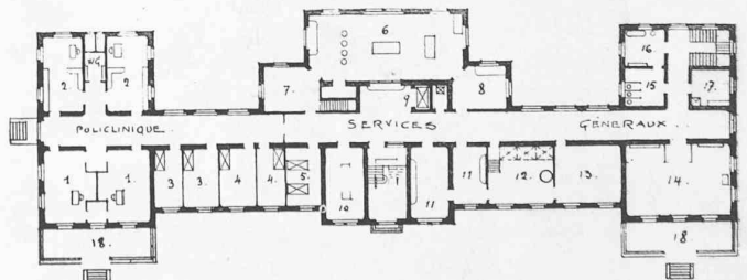
Bâtiment principal. Plan du rez-de-chaussée. — 1 : 800.
