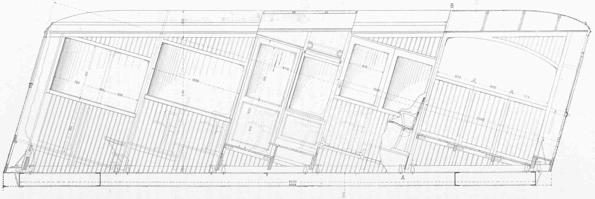
Fig. 11. — Voiture. — Plan et élévation. — 1 : 35.
