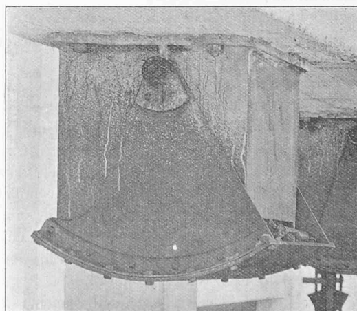
Fig. 47. — Trappe de reprise à coke.
