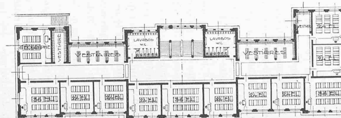
Plan du 2 me étage. — 1 : 800.
