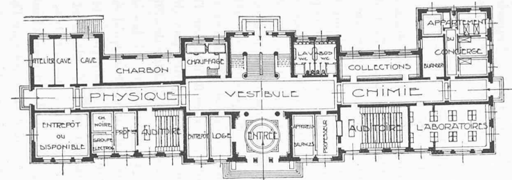
Plan du rez-de-chaussée inférieur. — 1 : 800.
