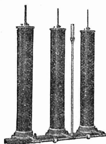
Résistance liquide.
