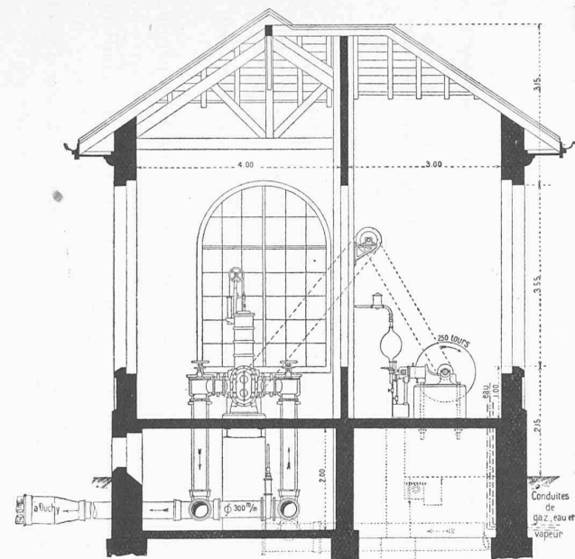
Fig. 17. — Coupe transversale.
