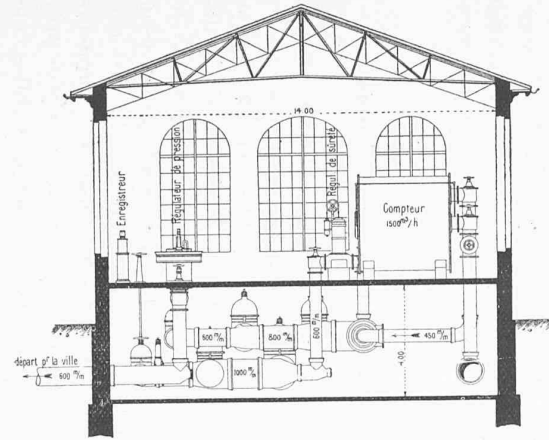
Fig. 22. — Coupe transversale.
