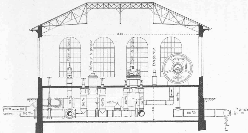
Fig. 21. — Coupe longitudinale.
