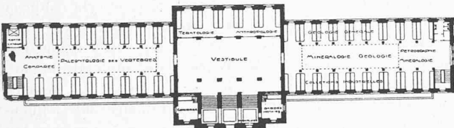
Rez-de-chaussée. — 1 : 1200.
