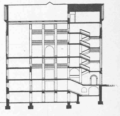
Coupe transversale.
