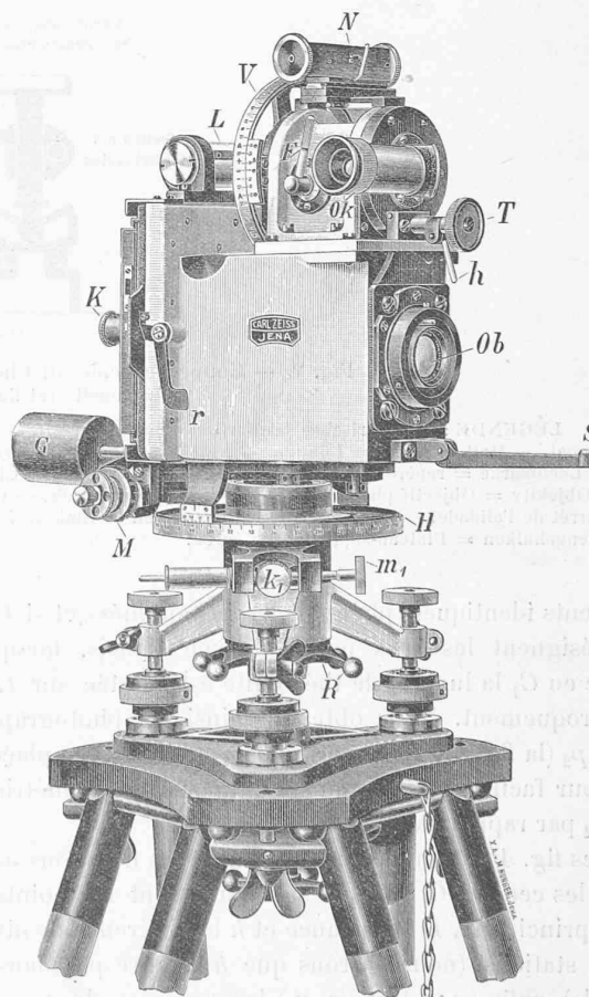
Fig 1. — Photothéodolite Zeiss. Modèle B ( \frac{1}{5} grandeur naturelle) les deux appareils à objectif fixe et munis de cercles donnant la minute.
