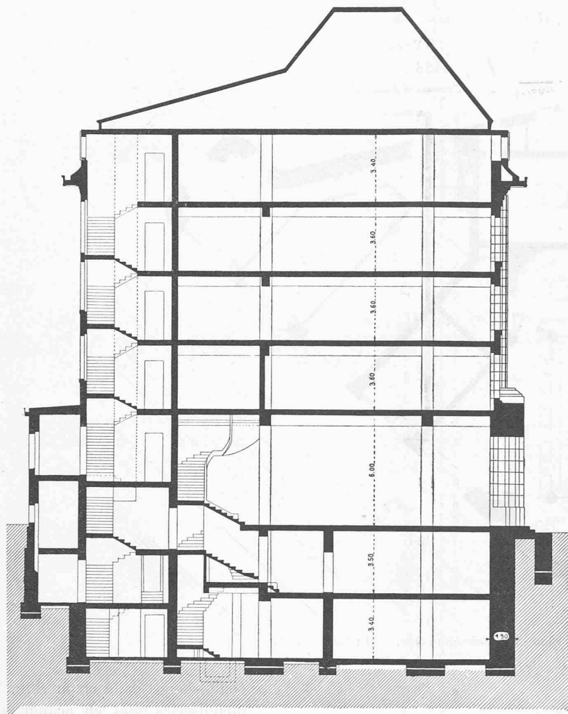
Coupe. — 1 : 250.
