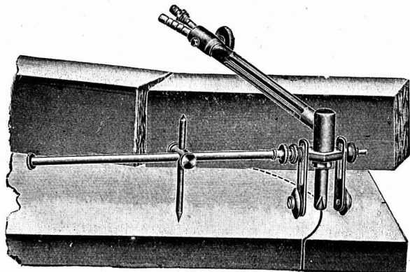
Chalumeau combiné « Universel »
