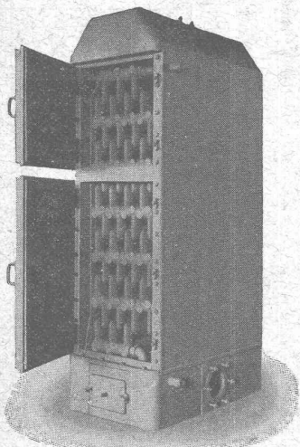
Calorifère récupérateur breveté
