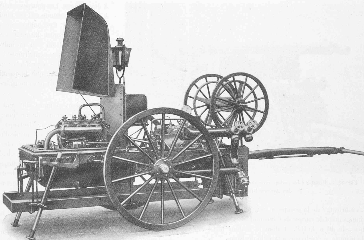
Fig. 20. — Pompe à incendie à bras à deux roues, avec moteur de la maison Arbenz.
