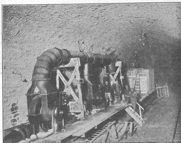
Relais de ventilation au km. 1,850.
