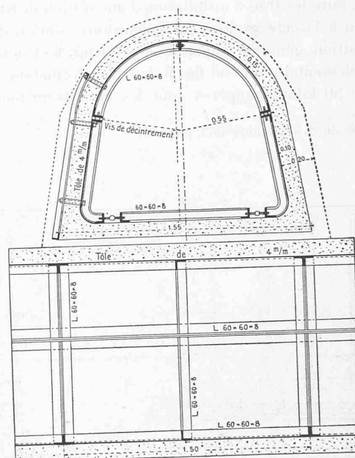
Fig. 17. — Conduite. — 1 : 300.
