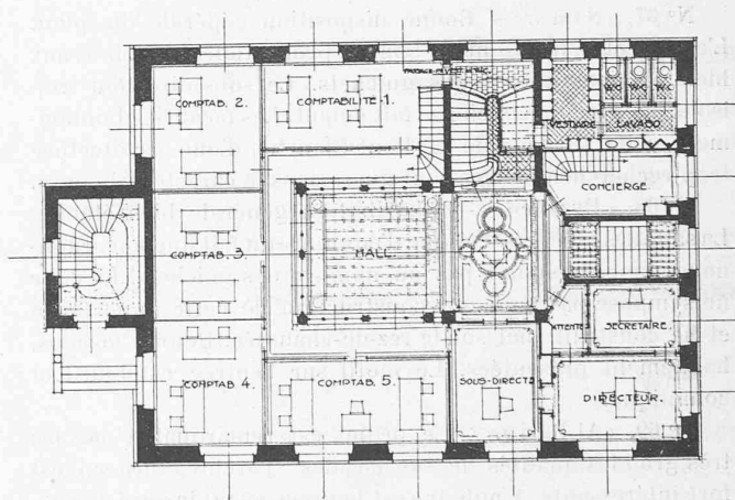
Plan du rez-de-chaussée. — 1 : 300.
