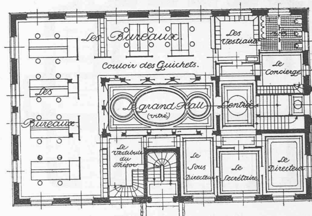
Plan du rez-de-chaussée. — 1 : 300.
