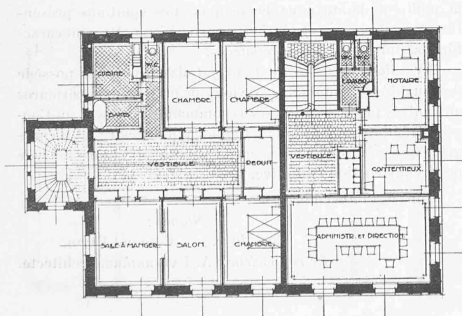
Plan du premier étage. — 1 : 300.
