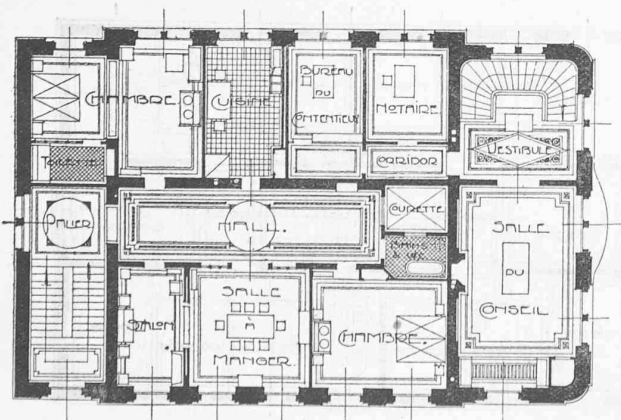
Plan du 1 er étage. — 1 : 300.
