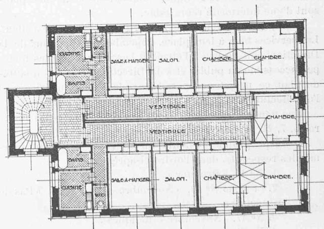
Plan du deuxième étage. — 1 : 300.
