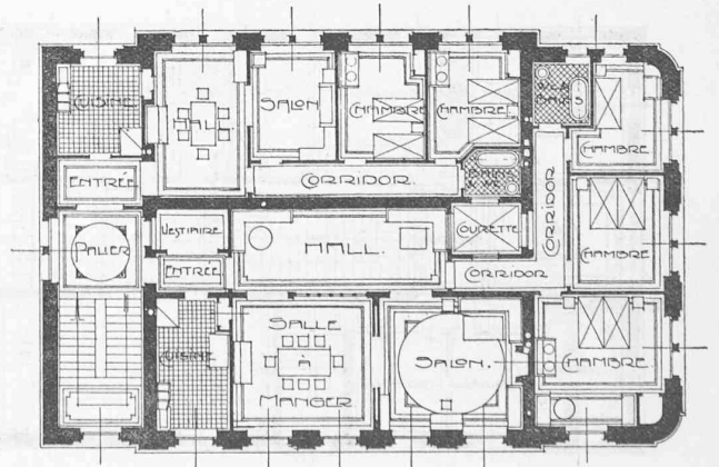
Plan du 2 me étage. — 1 : 300.
