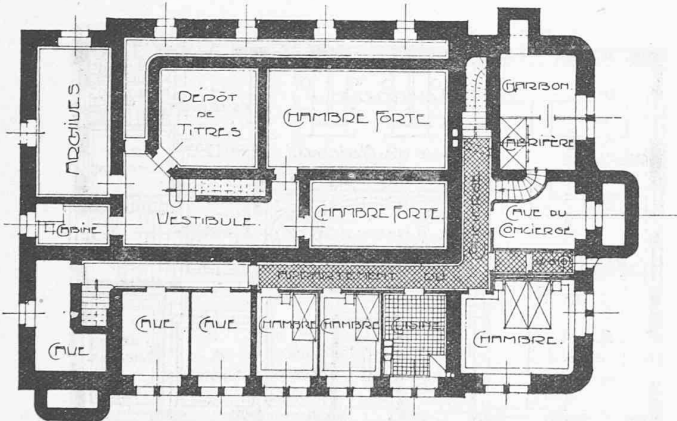
Plan du sous-sol. — 1 : 300.
