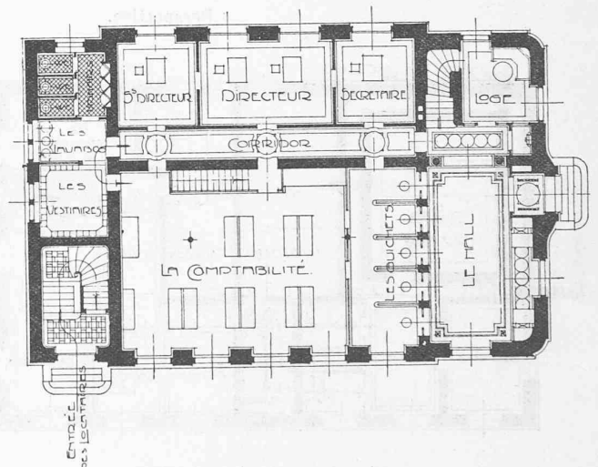
Plan du rez-de-chaussée. — 1 : 300.
