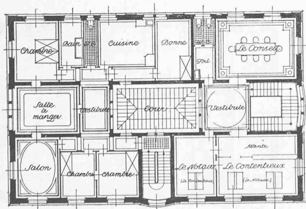
Plan du premier étage. — 1 : 300.
