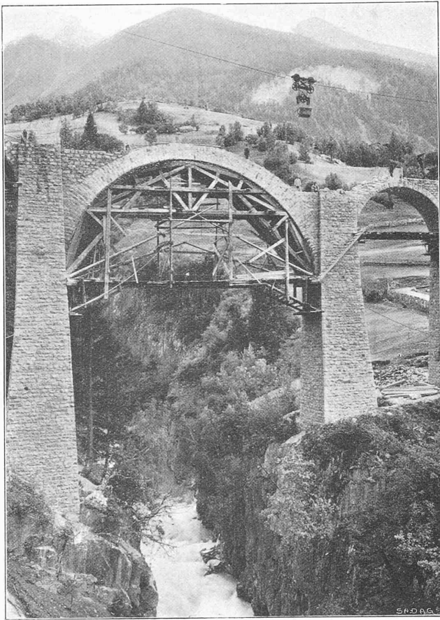
Fig. 14. — Le viaduc de Grenchiols.
