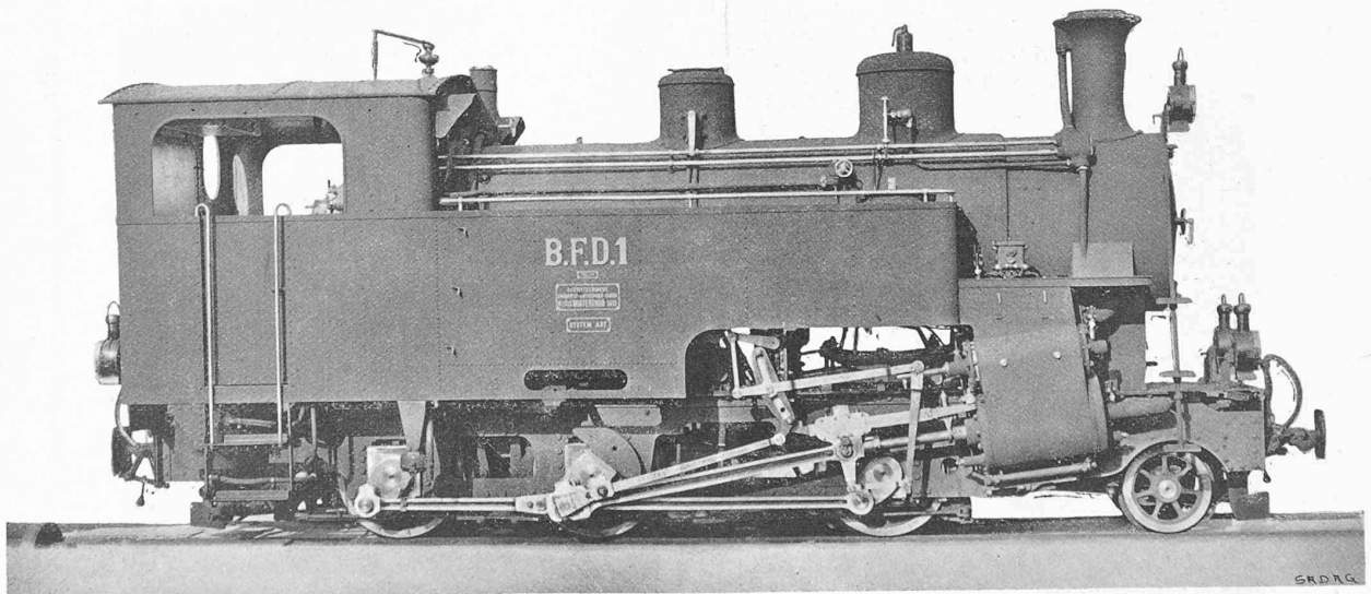
Fig. 17. — Locomotive à crémaillère tournie par la Société suisse pour la construction de locomotives et de machines, à Winterthur.
