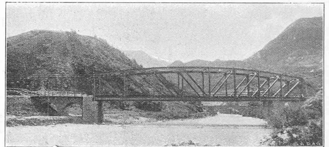
Fig. 16. — Le pont sur la Massa.
