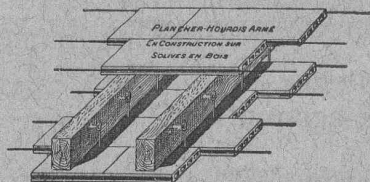
Plafond-hourdis armé s/solives en bois.
